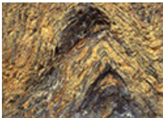
Schistus_Schist.jpeg
